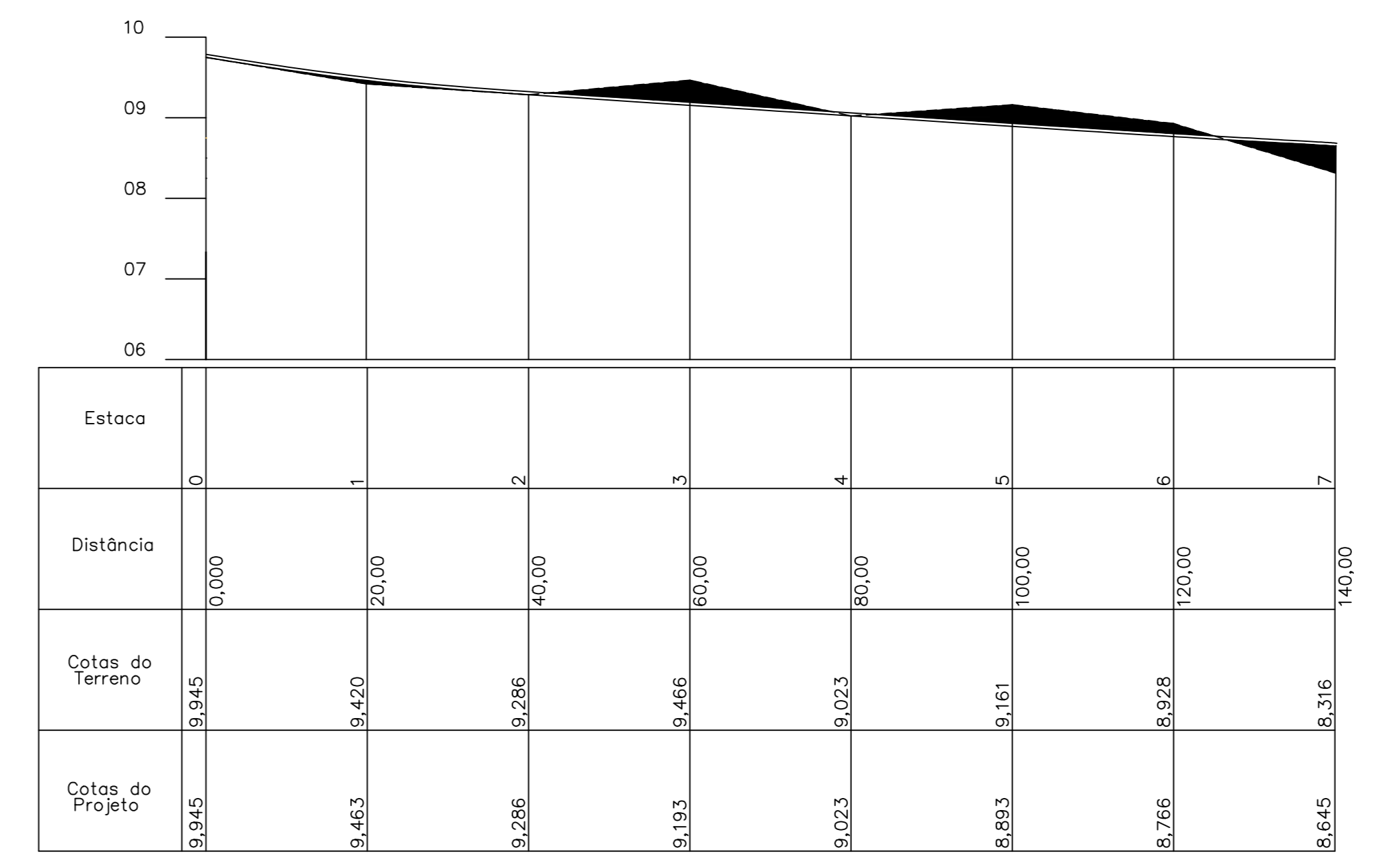
PERFIL LONGITUDINAL-RUA PROJETADA 03 ESCALA HORIZONTAL 1:500 ESCALA VERTICAL 1:50
