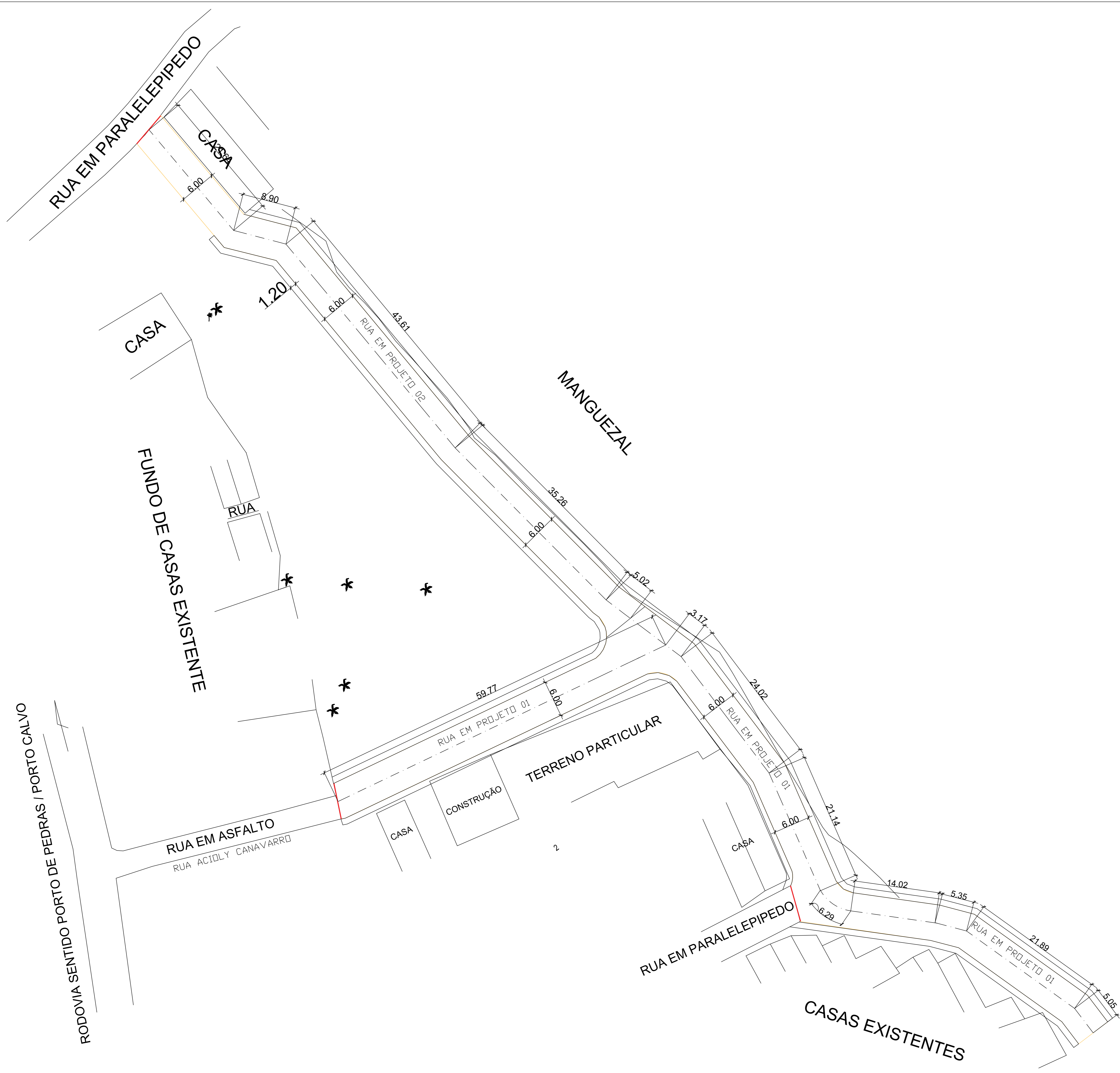
PLANTA BAIXA - COTADA ESCALA 1/200
